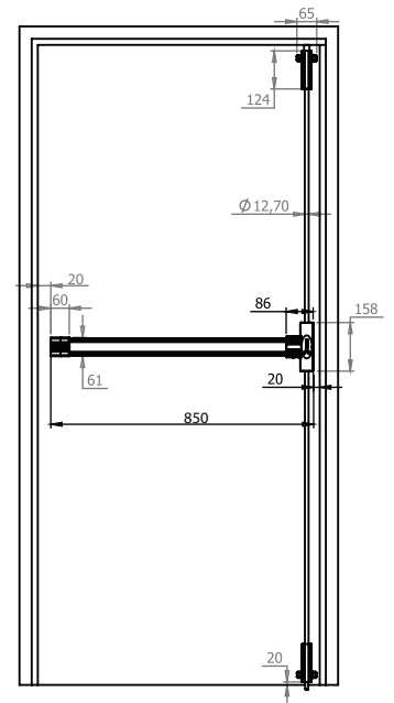
BARRA ANTIPÂNICO TOUCH VERTICAL
